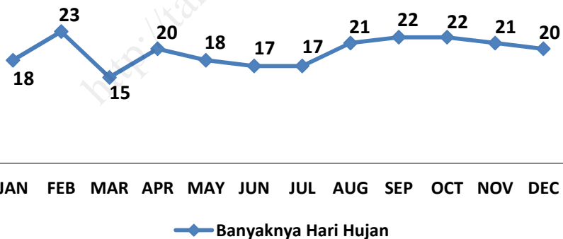
Grafik 1.2 Banyaknya Hari Hujan Menurut Stasiun Pondok Betung Kota Tangerang Selatan Tahun 2016
